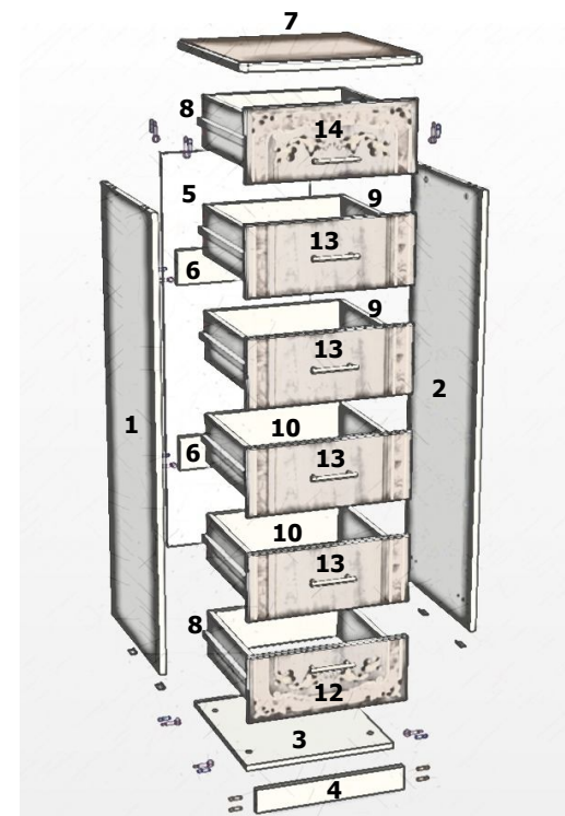
Паспорт и схема сборки
