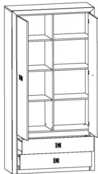
Шкаф REG2D2S выс./шир./глуб. 200.5/103.5/40 см
